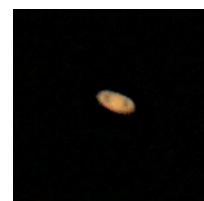
環のある土星ですが、ガリレオの望遠鏡では環とは認識できませんでした。
