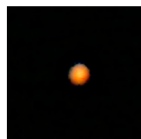
今年の夏大接近した火星。まだまだ明るく赤く輝いています。
